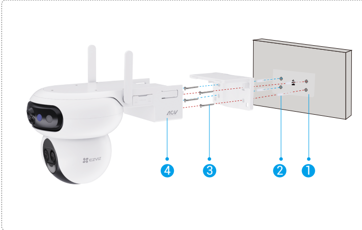
그림 2 벽 장착
