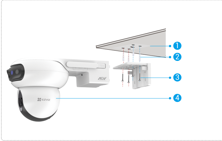
그림 1 천장 장착
